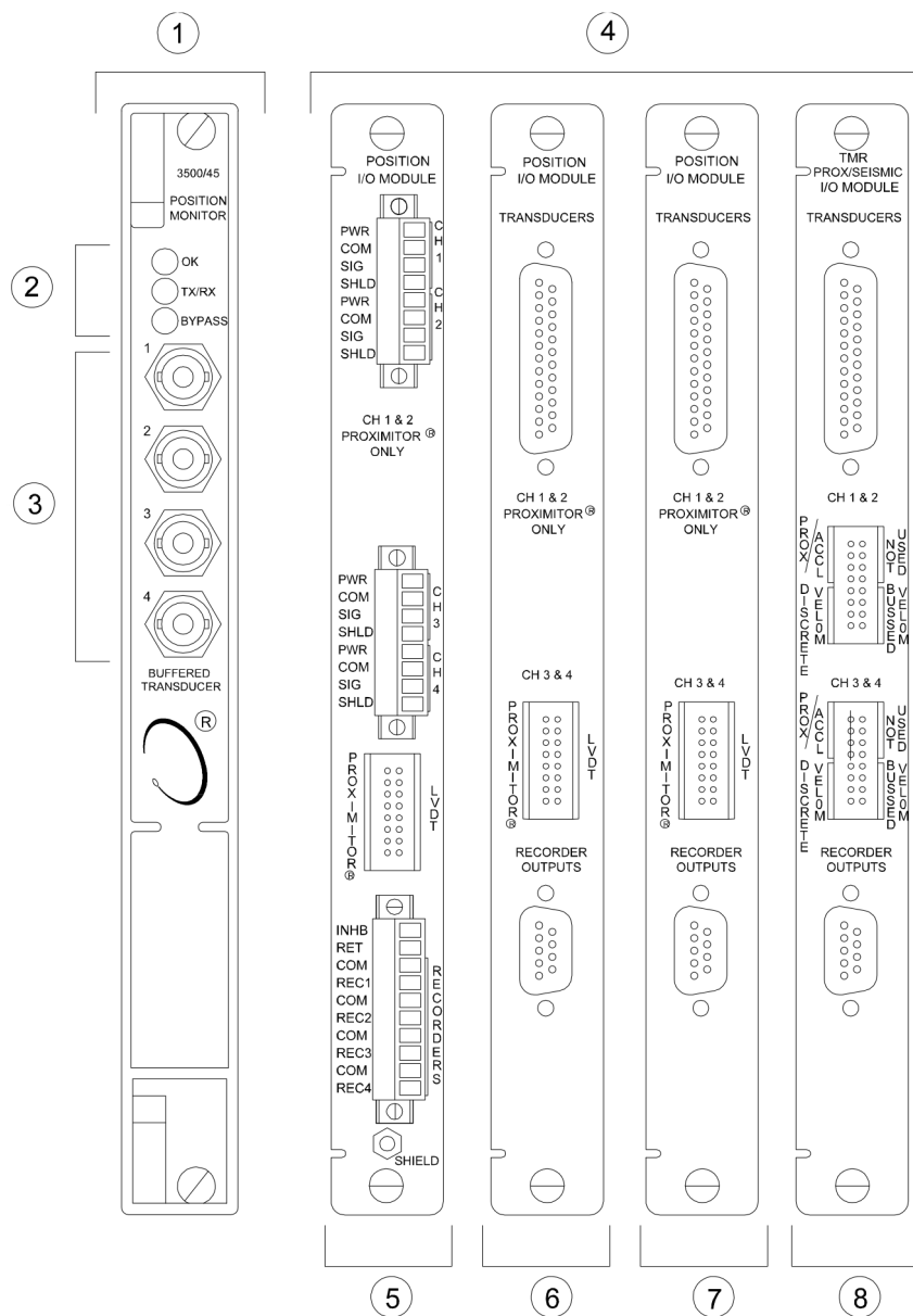
Рисунок 1: Монитор положения (вид спереди); модули ввода/вывода (вид сзади) для датчиков Proximitor, датчика положения и ЛДТ постоянного тока.
